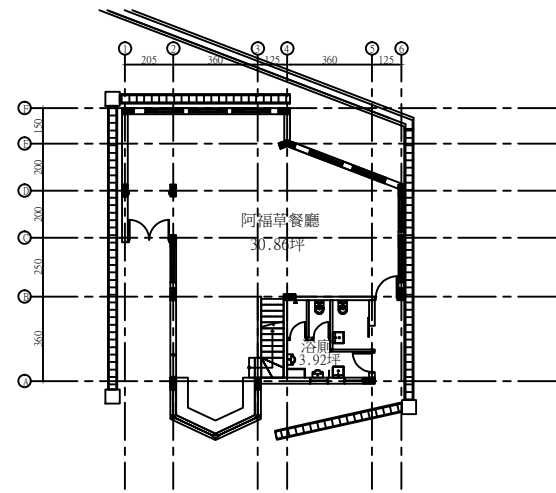
一樓平面圖
