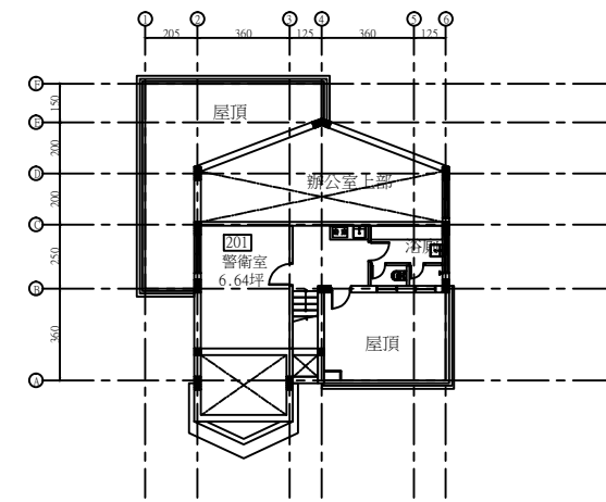
二樓平面圖
