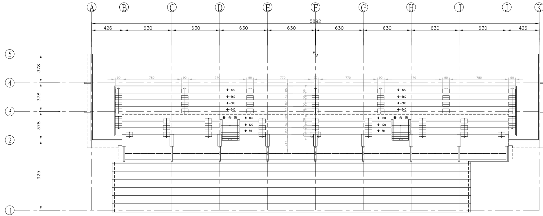
看台層平面圖 SCALE : 1/100
