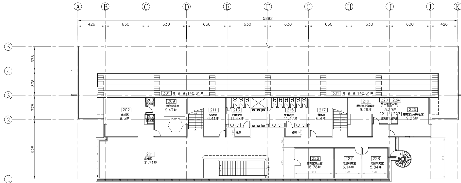
貳層平面圖 SCALE : 1/100
