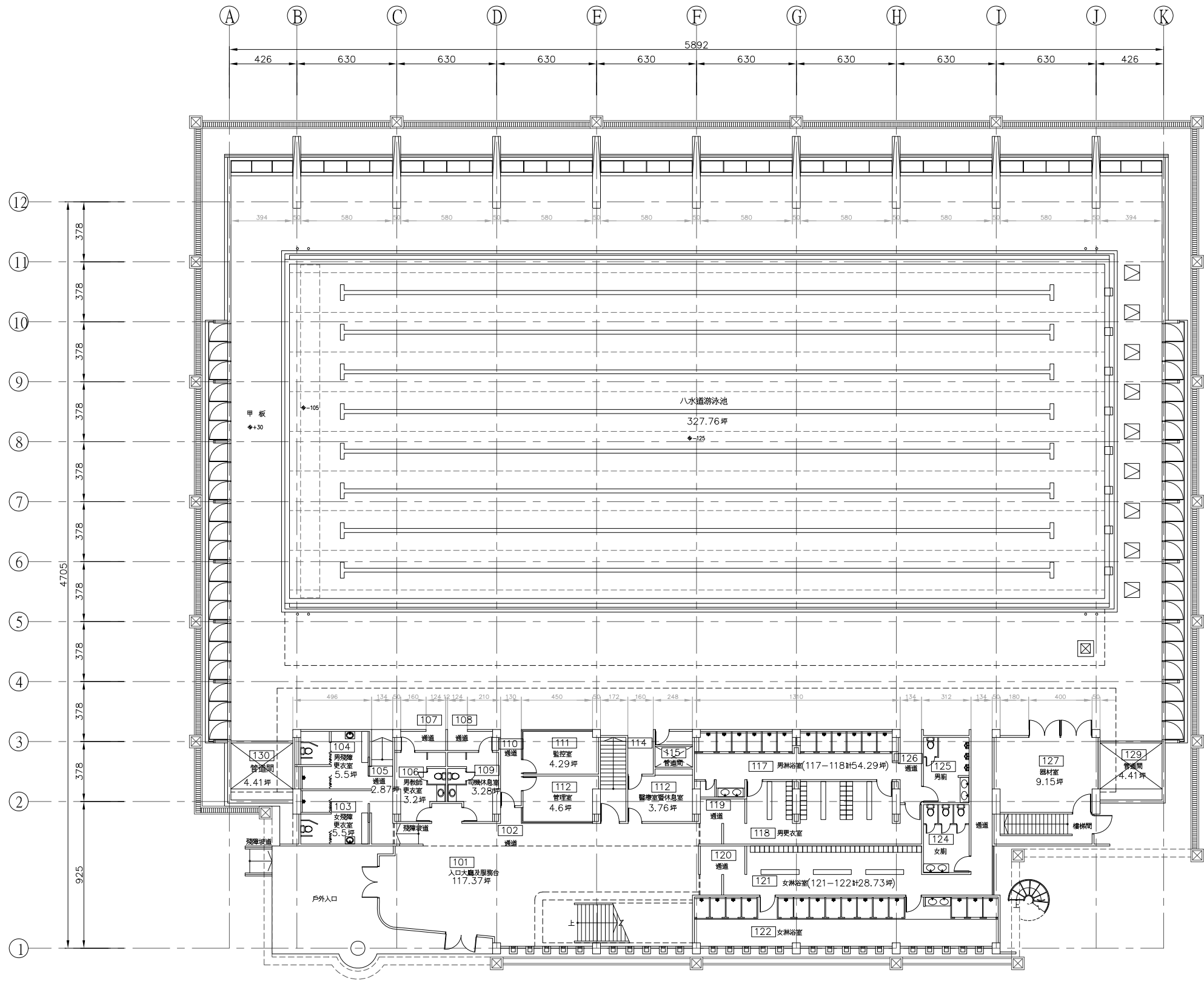
壹層平面圖 SCALE : 1/100
