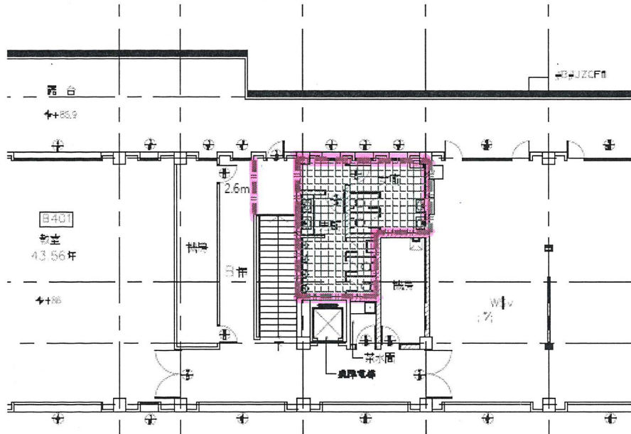
1 活動中心4F假設工程圖 UNIT: CM SCALE: A3=1/250
