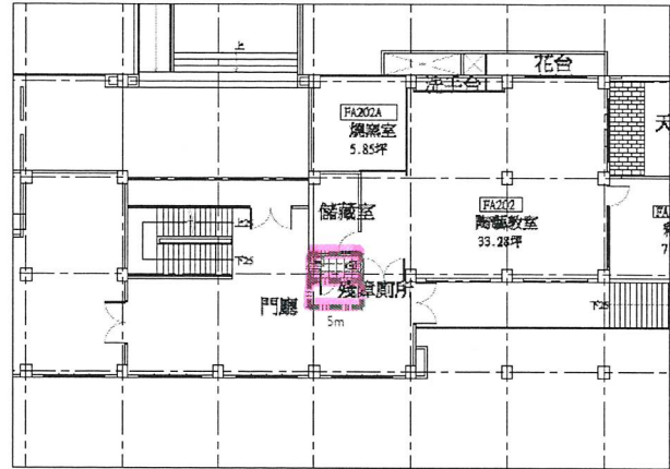
3 美術系特殊教室廁所2F假設工程圖 UNIT: CM SCALE: A3=1/250
