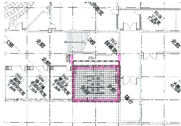
3 美術系後區2F假設工程圖 UNIT: CM SCALE: A3=1/250
