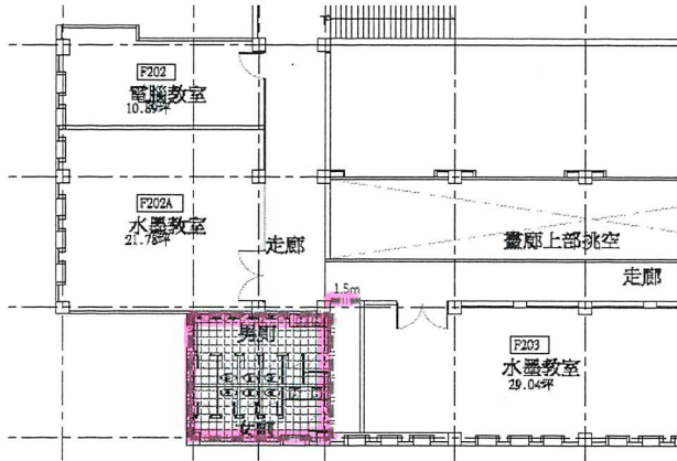
2 美術系前區2F假設工程圖 UNIT: CM SCALE: A3=1/250
